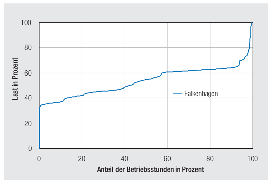
Abb. 4: Lastverteilung der Methanisierungsanlage Falkenhagen
