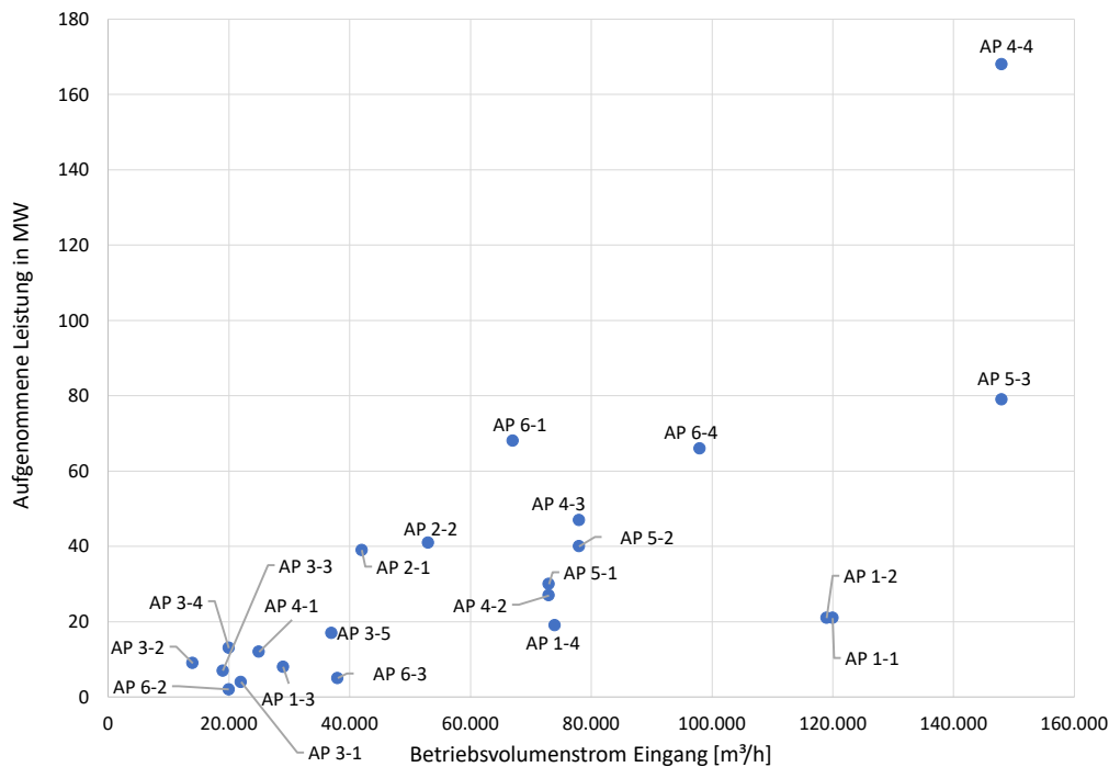
Abbildung 4.2. Aufgenommene Leistung.
