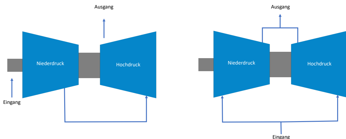
Abbildung 4.5. Back-to-Back-Anordnung.
